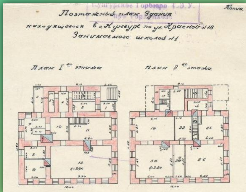
Поэтажный план здания школы №1, 1950-е гг. Р-176, оп.1, д.376
