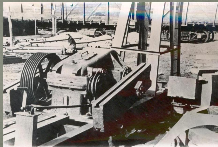
Редукторный станок СКН - 5. Изготавливался заводом с 1943 года, БФ. д.820
